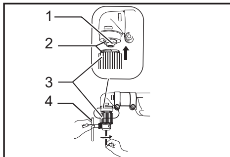
► 1. Eje 2. Dos caras 3. Mandril de taladro 4. Llave de mandril
