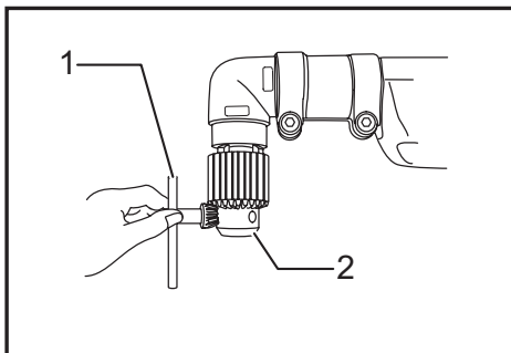
► 1. Clé de mandrin 2. Mandrin
