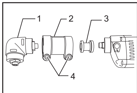
► 1. Caja angular 2. Junta 3. Dado 4. Tornillo
