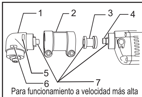
► 1. Caja angular 2. Junta 3. Dado 4. Eje 5. Baja 6. Alta 7. Dos caras
