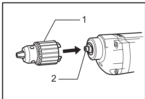
► 1. Mandril de taladro 2. Eje
