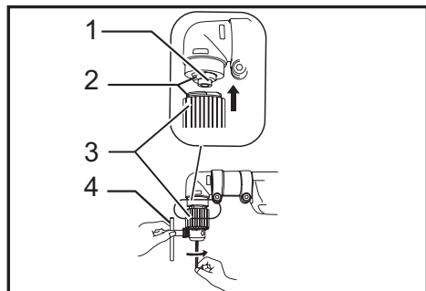
► 1. Axe 2. Deux faces 3. Mandrin 4. Clé de mandrin
