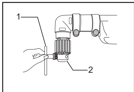
► 1. Llave de mandril 2. Mandril de taladro
