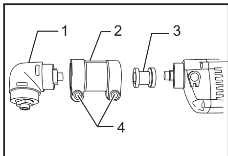
► 1. Carter d'angle 2. Raccord 3. Douille 4. Boulon
