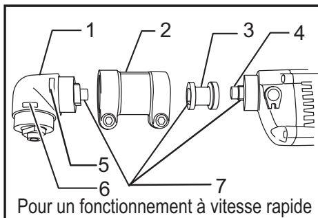
► 1. Carter d'angle 2. Raccord 3. Douille 4. Axe 5. Réduite 6. Grande 7. Deux faces
